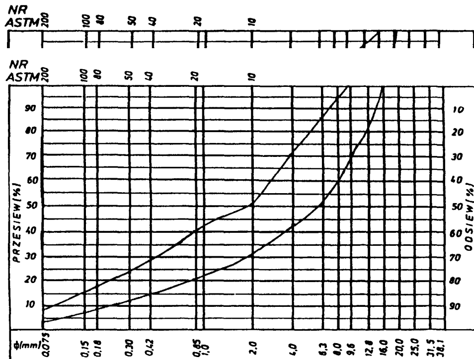
Rys. 8. Krzywe graniczne uziarnienia mieszanek mineralnej 0+20 mm do warstwy wiążącej, wyrównawczej i wzmacniającej
