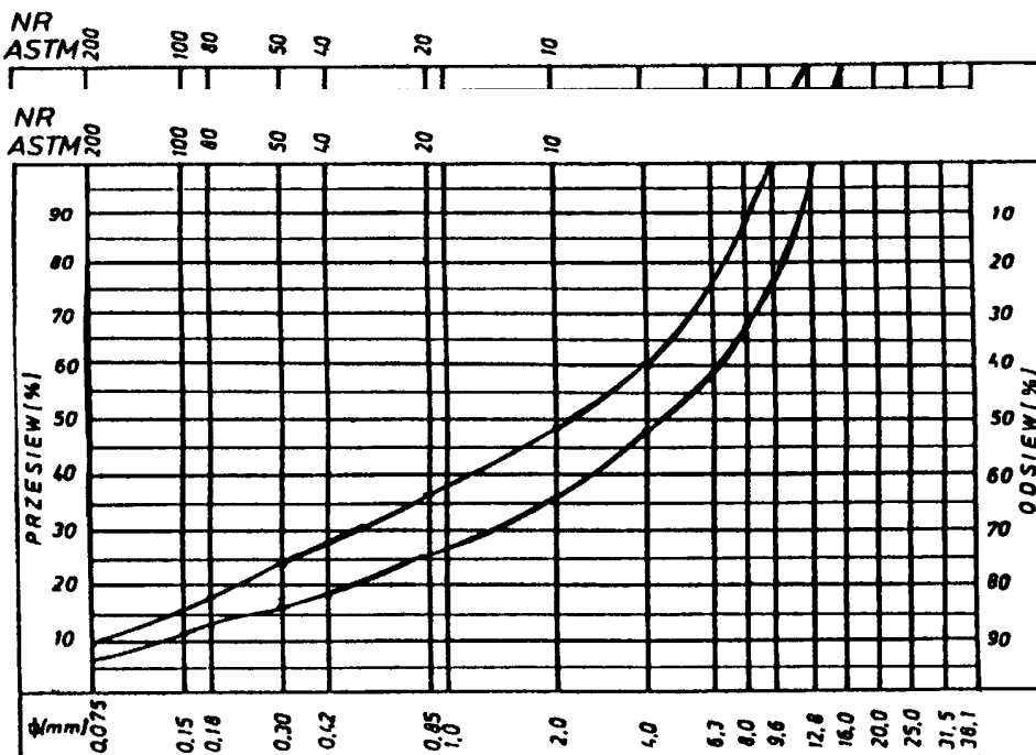
Rys. 6. Krzywe graniczne uziarnienia mieszanki mineralnej 0+16 mm do warstwy ścieralnej z betonu
