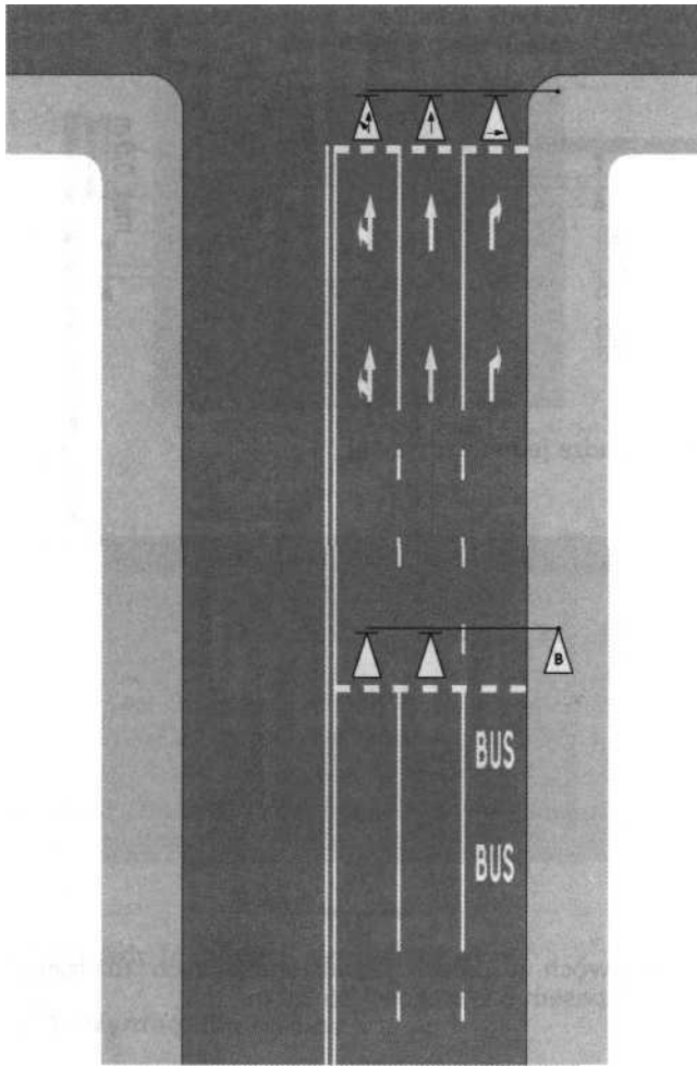
Rys. 7.3.2. Zasada lokalizacji sygnalizatorów dla pojazdów komunikacji publicznej umożliwiających im wyjazd z wydzielonego dla nich pasa ruchu (śluza)
